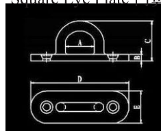
Square Eye Plate 门鼻子
