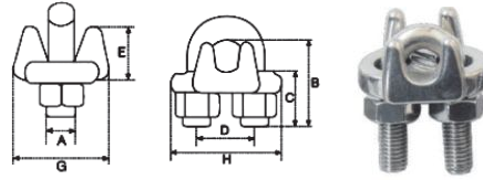
US TYPE WIRE ROPE CLIPS 美式模锻卡头
