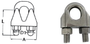
WIRE ROPE CLIP DIN741 卡头
