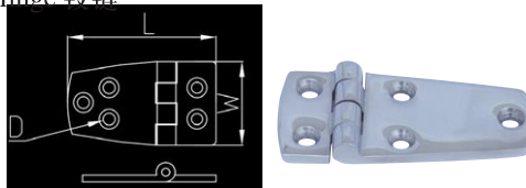
Hinge 铰链
