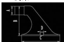
Stanchion 支架
