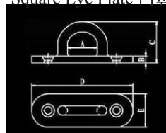
Square Eye Plate 门鼻子
