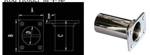
Rod Holder 鱼竿座
