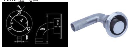
Tank Vent 透气口
