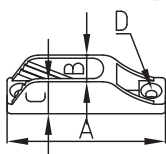
Cleats Inox For Ropes 3/6 mm 夹绳器
