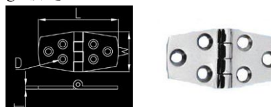
Hinge 铰链
