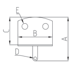
Hinge 铰链
