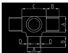
Tees 四通
