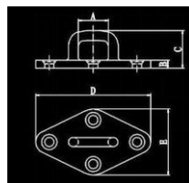
Square Eye Plate 门鼻子
