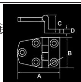
Hinge 铰链
