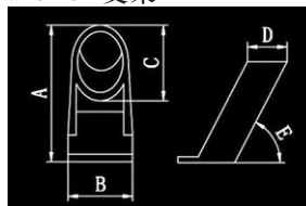
Stanchion 支架
