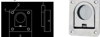
Lift Ring 地板扣
