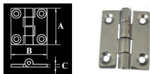
Hinge 铰链
