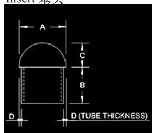
Insert 塞头
