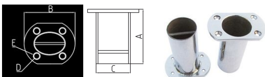
Rod Holder 鱼竿座
