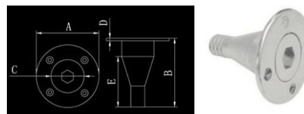
Deck Filler 加油口
