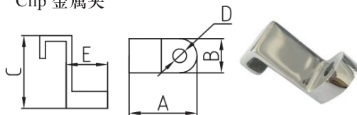
Clip 金属夹
