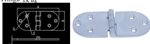
Hinge 铰链
