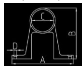
Stanchion(Center) 船中支架
