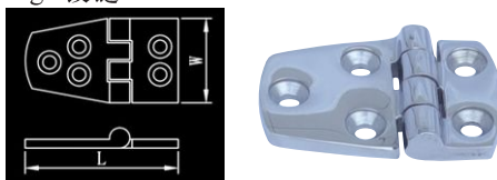
Hinge 铰链
