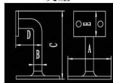
Stanchion 支座
