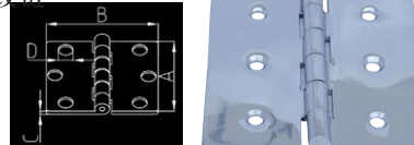
Hinge 铰链
