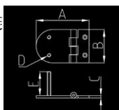
Hinge 铰链
