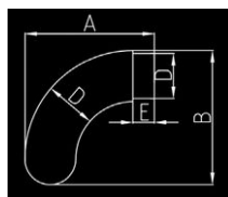
Insert 塞头
