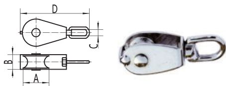
PULLEY 犁形单滑轮
