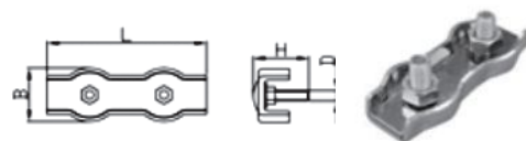
DUPLEX WIRE ROPE CLAMP 卡座
